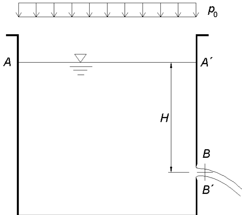
Slika 4.1 Istjecanje kroz mali otvor u vertikalnoj stjenci
