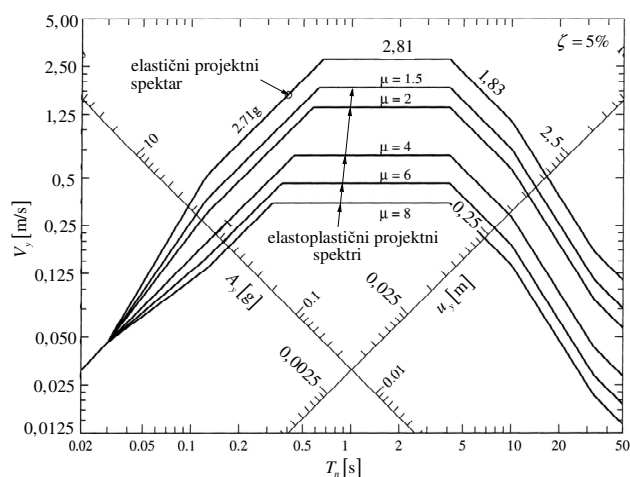
Slika 149.: Elasto-plastični spektra odziva (fraktila: 84,1 %) za različite koeficijente duktilnosti \mu i \zeta=0,05
