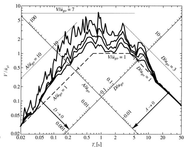
Slika 118.: Normirani D - V - A spektar za potresni zapis El Centro, uz prigušenja 0, 2, 5 i 10%
