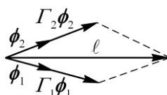
Slika 213.: Raspis utjecajnoga vektora po oblicima titranja
