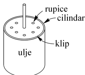
Slika 15.: Viskozni prigušivač
