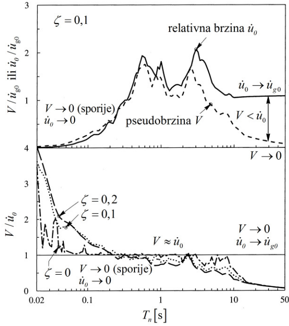
Slika 140.: Usporedba spektara odziva pseudobrzine i relativne brzine, \zeta=0,1 ; omjer spektara V/\ddot{u}_0 za različita prigušenja
