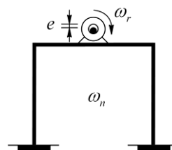
Slika 74.: Pobuda turbinskog stola ekscentričnom masom turbine
