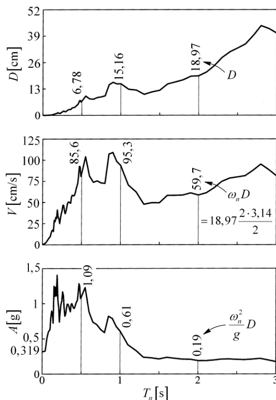
Slika 111.: Spektri odziva za potresni zapis El Centro: pomaka, pseudobrzine i pseudoubiranja, za \zeta=0,02
