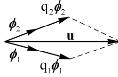
Slika 192.: Raspis vektora pomaka po vlastitim vektorima
