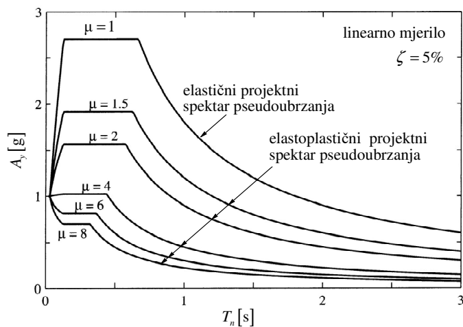
Slika 150.: Elasto-plastični projektni spektri (fraktila: 84,1 %) potresnih zapisa s \ddot{u}_{g0} = 1g , \dot{u}_{g0} = 1,22\text{m/s} , u_{g0} = 0,91\text{m} , za različite koeficijente duktilnosti \mu i \zeta=0,05
