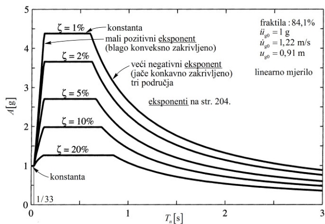
Slika 135.: Elastični projektni spektri pseudoubrzanja (fraktila: 84,1%) potresnih zapisa s \ddot{u}_{g0} = 1 g , \dot{u}_{g0} = 1,22 m/s , u_{g0} = 0,91 m , za različita prigušenja
