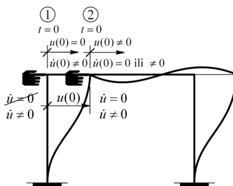
Slika 45.: Objašnjenje početnih uvjeta na okviru
