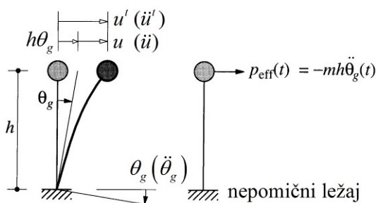
Slika 36.: Efektivna sila potresa za rotacijsku potresnu pobudu
