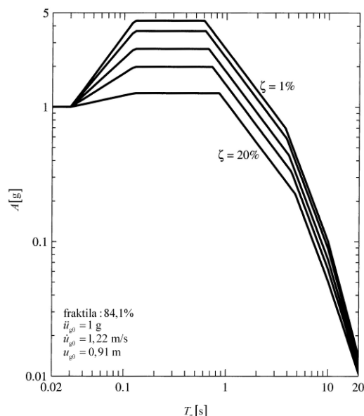
Slika 134.: Elastični projektni spektri pseudoubrzanja (fraktila: 84,1%) potresnih zapisa s \ddot{u}_{g0} = 1 g , \dot{u}_{g0} = 1,22 m/s , u_{g0} = 0,91 m , za različita prigušenja
