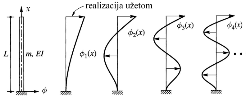
Slika 198.: Vlastiti oblici titranja konzole
