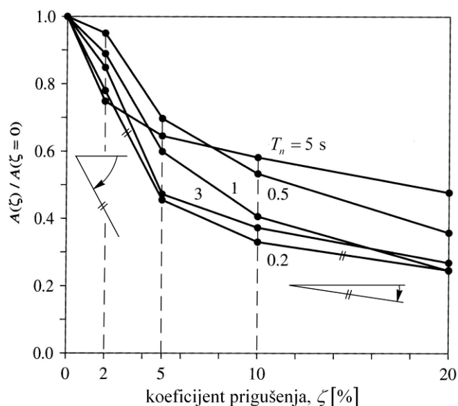
Slika 124.: Promjene vršnog pseudoubrzanja u odnosu na prigušenje za različite sustave s jednim stupnjem slobode; potresni zapis El Centro
