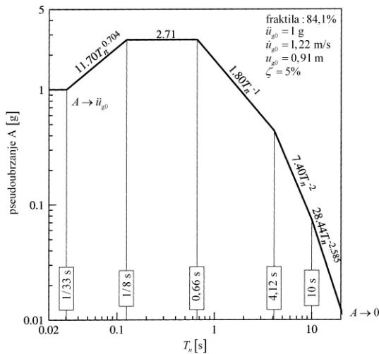
Slika 131.: Elastični projektni spektar pseudobrzanja (fraktila: 84,1%) potresnih zapisa za \ddot{u}_{g0} = 1g , \dot{u}_{g0} = 1,22\text{ m/s} , u_{g0} = 0,91\text{ m} , uz \zeta=0,05
