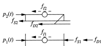
Slika 163.: Ravnoteža sila posmičnoga okvira
