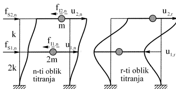
Slika 191.: Dvokatni posmični okvir: n -ti i r -ti oblik titranja
