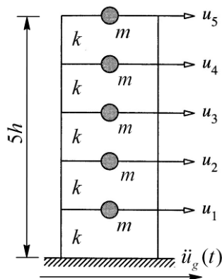
Slika 220.: Model peteroetažne posmične zgrade
