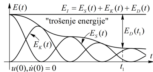
Slika 60.: Energija slobodnog titranja uz prigušenje
