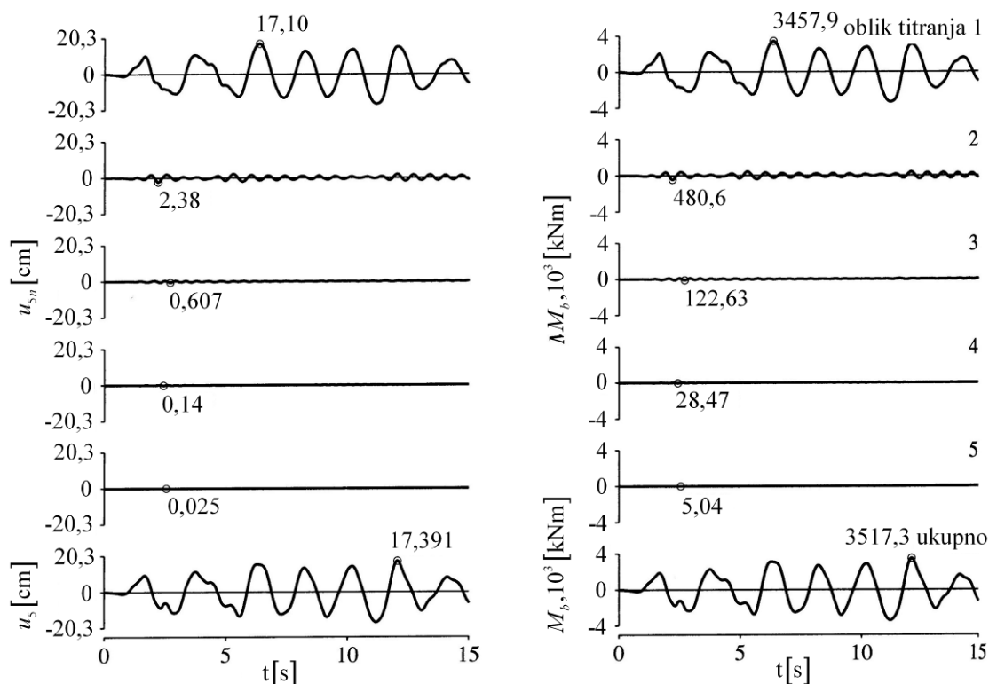
Slika 226.: Pomak krova i moment prevrtanja poopcénog sustava i ukupni odzivi
