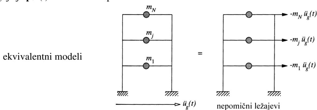
Slika 180.: Efektivne sile potresa
