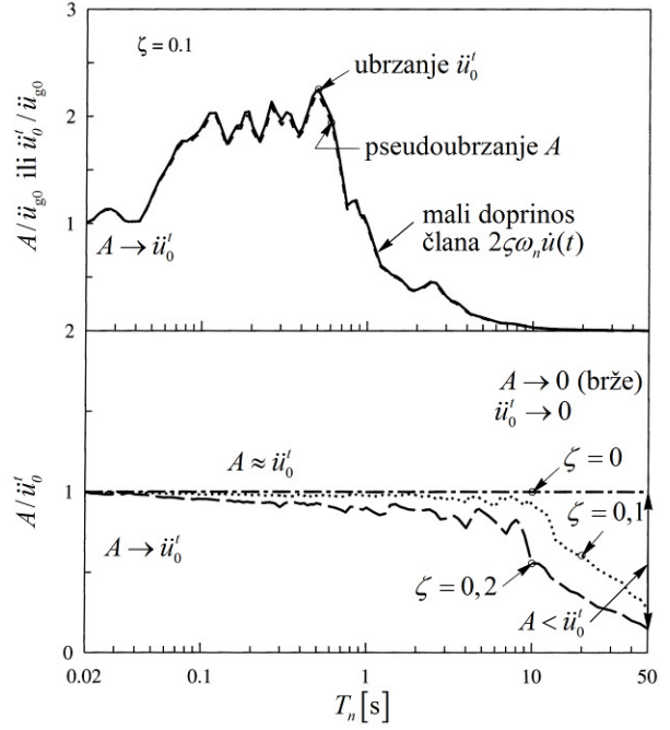
Slika 141.: Usporedba spektara odziva pseudoubznanja i ukupnog ubrzanja, \zeta=0,1 ; omjer spektara A/\ddot{u}_0' za različita prigušenja
