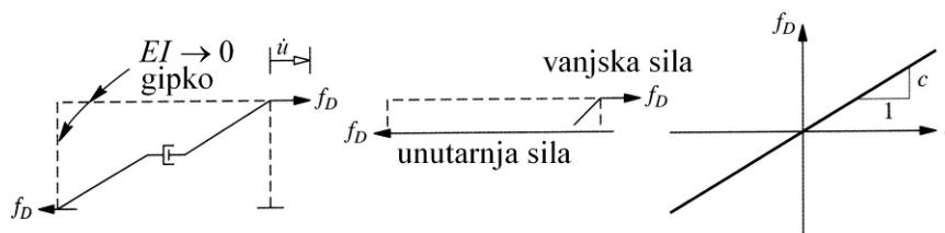
Slika 26.: Ponašanje linearnog viskoznog prigušivača
