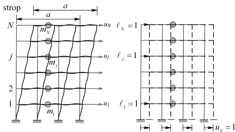
Slika 215.: Bočni pomaci višeetažnog okvira zbog translacijske pobude potresom
