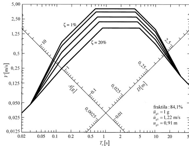
Slika 133.: Elastični projektni spektri pseudobrzine (fraktila: 84,1%) potresnih zapisa za \ddot{u}_{g0} = 1g , \dot{u}_{g0} = 1,22\text{ m/s} , u_{g0} = 0,91\text{ m} , za različita prigušenja
