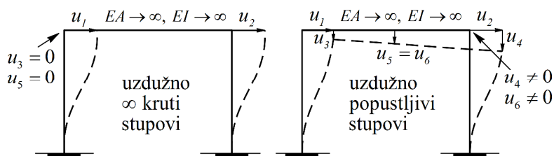
Slika 178.: Uzdužno \infty kruti i uzdužno popustljivi stupovi
