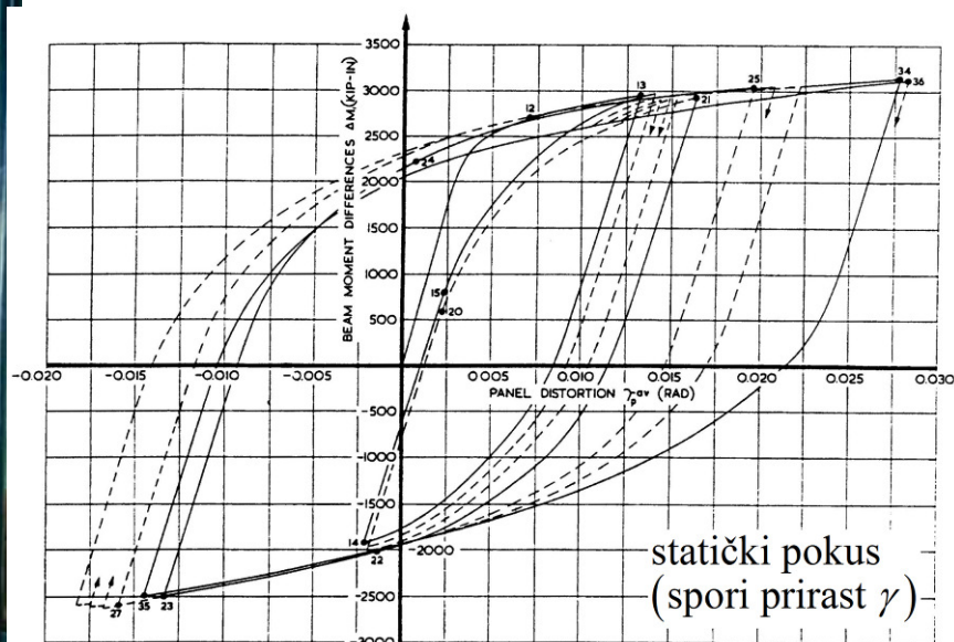
Slika 24.: Odnos sila-deformacija za čelični konstruktivni element
