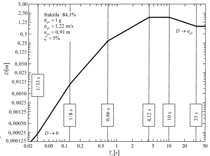
Slika 132.: Elastični projektni spektar pomaka (fraktila: 84,1%) potresnih zapisa za \ddot{u}_{g0} = 1g , \dot{u}_{g0} = 1,22\text{ m/s} , u_{g0} = 0,91\text{ m} , uz \zeta=0,05
