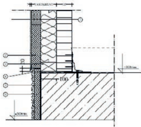
Slika 2-83 Drveni masivni zid, žbukana fasada [211]
