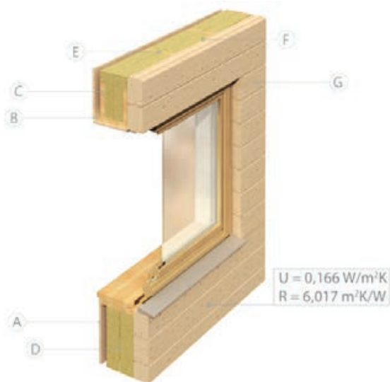
Detalj spoja ugradnje prozora u vanjski zid (izolacija s unutarnje strane)
