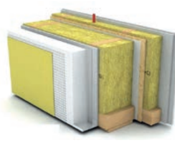
Sistem Mega d=45,8 U=0,093 W/m 2 K
