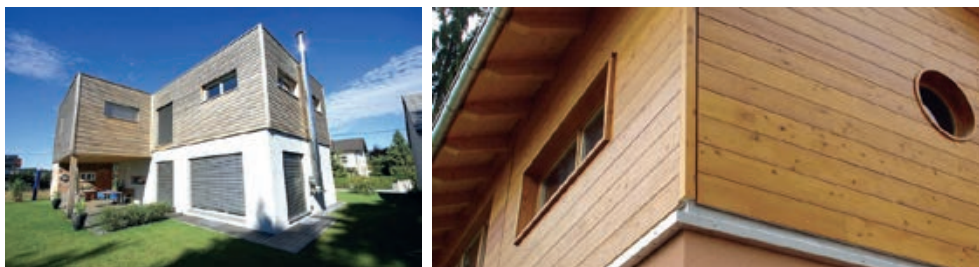
Slika 3-84 Detalj i fotografije prijelaza s ventilirane fasade na ETICS sustav [246], [245], [284]
