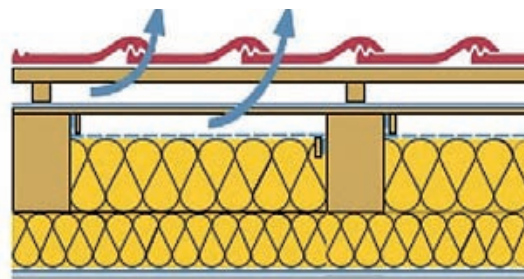
Slika 3-164 Primjer ventilacije u slučaju izvođenja krova s bitumenskom ljepenkom kao sekundarnim pokrovom [309]
