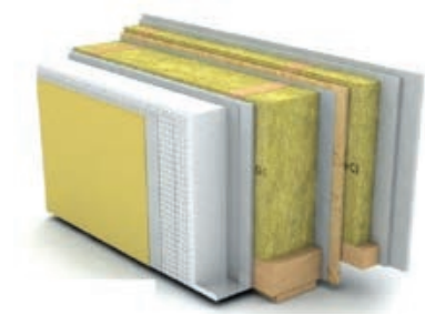
Sistem Euro d=36,8 U=0,118 W/m 2 K
