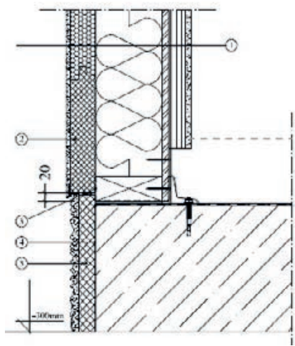
Slika 2-87 Drveni okvirni zid, žbukana fasada [211]
