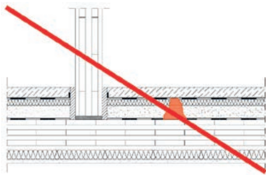
Slika 2-79 Shematski prikaz pojave zvučnog mosta u slučaju loše izvedene PE folije [210]
