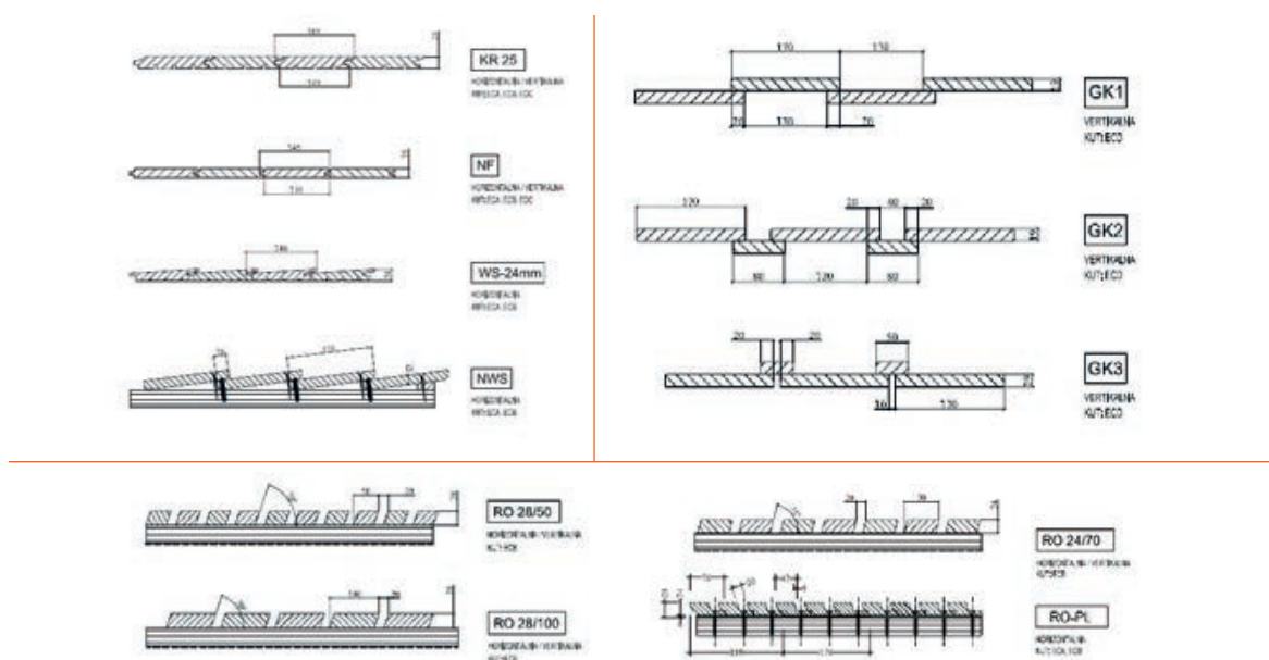
Slika 3-73 Tipovi drvenih fasada od dasaka i letvica [224]
