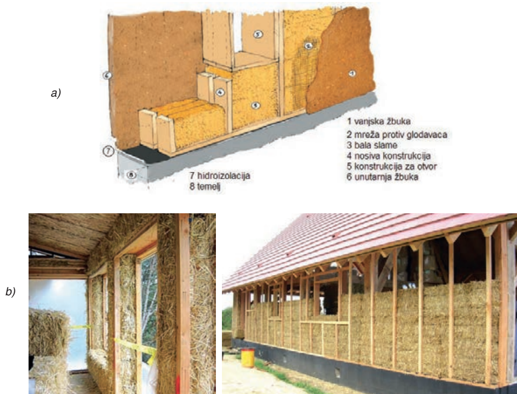
Slika 4-12 Zid od bala slame sa svim dijelovima na spoju s temeljem: a) crtež detalja s opisom slojeva; b) fotografije takvih zidova [346], [367], [368]
