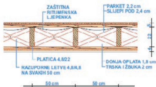
Slika 3-112 Drveni strop od platica [192]
