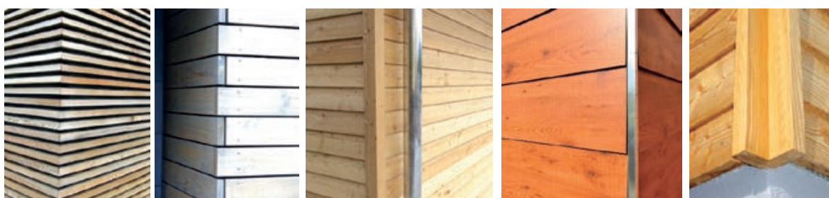
Slika 3-77 Fotografije nekih oblika kutnih završetaka [67], [276], [277], [278]
