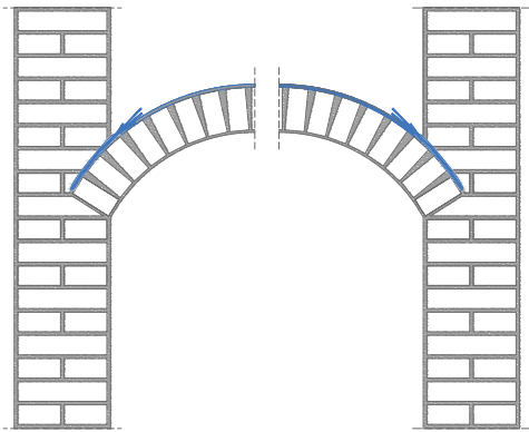
SIDRENJE VOLTE
