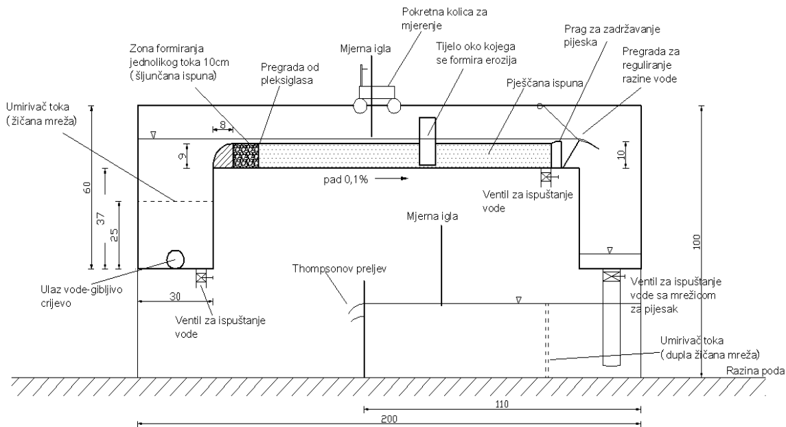
Slika 14.2 Hidraulička shema modela
