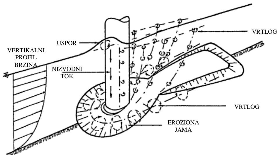
Slika 14.1 Opstrujavanje oko stupa kružnog poprečnog presjeka ( Raudkivi, 1998)
