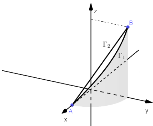
Slika 5.5: Krivulja \vec{\Gamma}
