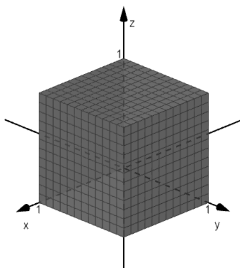
Slika 6.34: Kocka \Omega
