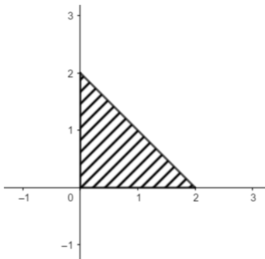
Slika 6.29: Projekcija D
