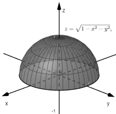
Slika 3.17: Tijelo \Omega
