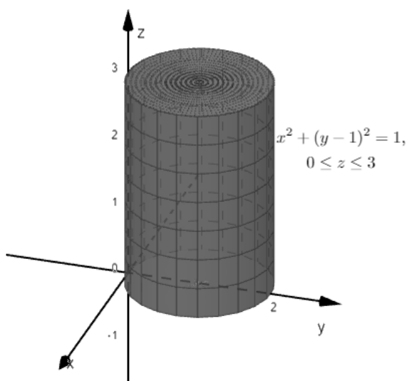
Slika 3.24: Tijelo \Omega
