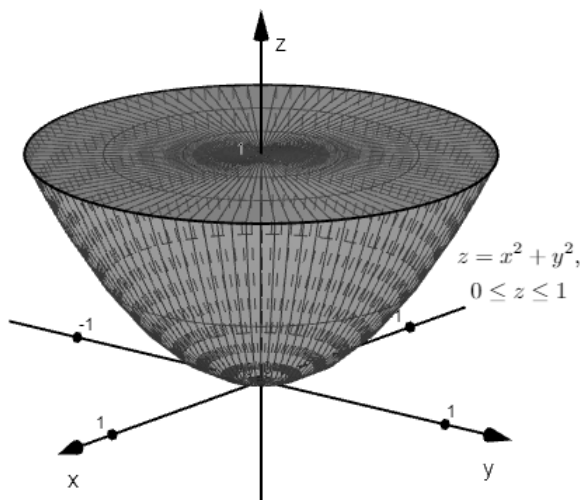
Slika 3.23: Tijelo \Omega
