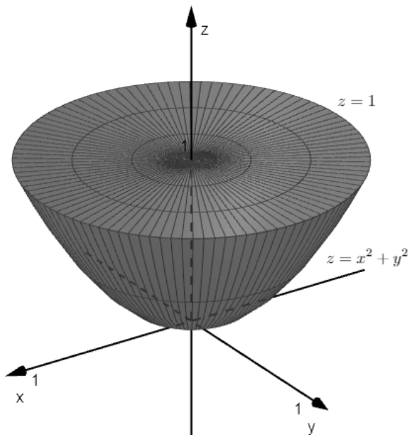
Slika 6.36: Ploha \vec{\Sigma}
