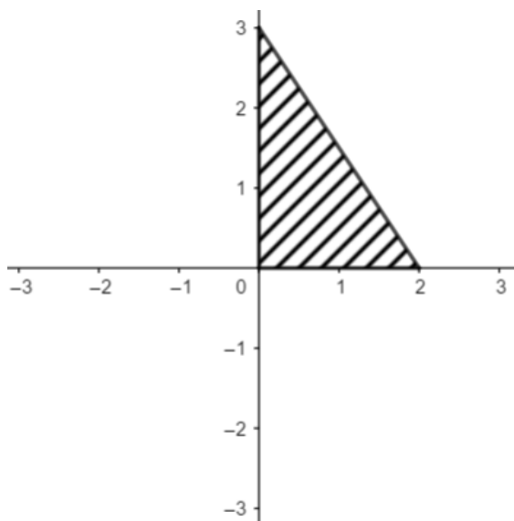
Slika 6.4: Projekcija D na xy -ravninu
