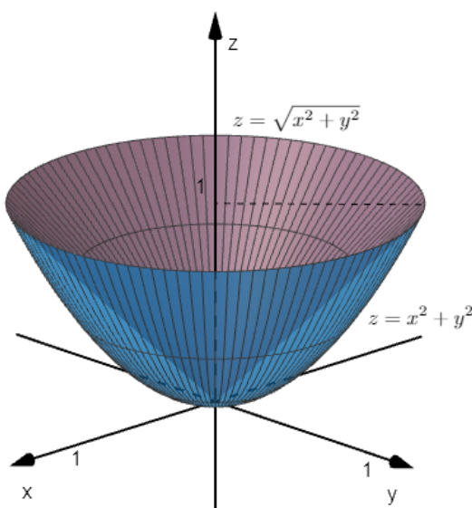
Slika 6.37: Ploha \vec{\Sigma}
