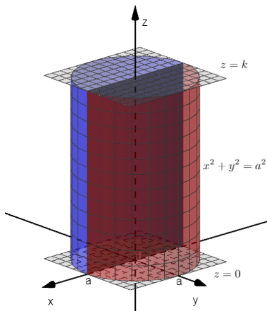
Slika 6.23: Ploha \Sigma
