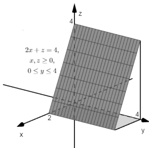
Slika 6.30: Ploha \vec{\Sigma}
