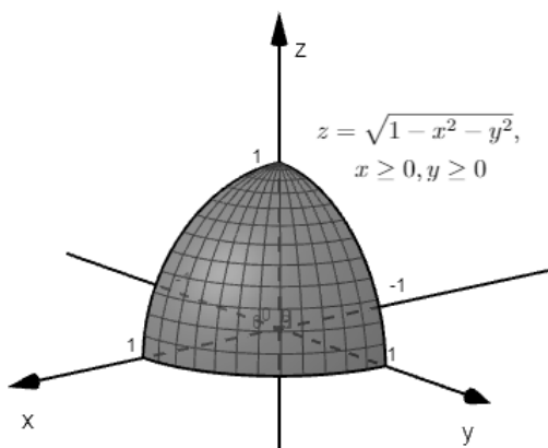
Slika 3.18: Područje integracije
