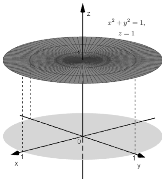
Slika 6.38: Ploha \vec{\Sigma}
