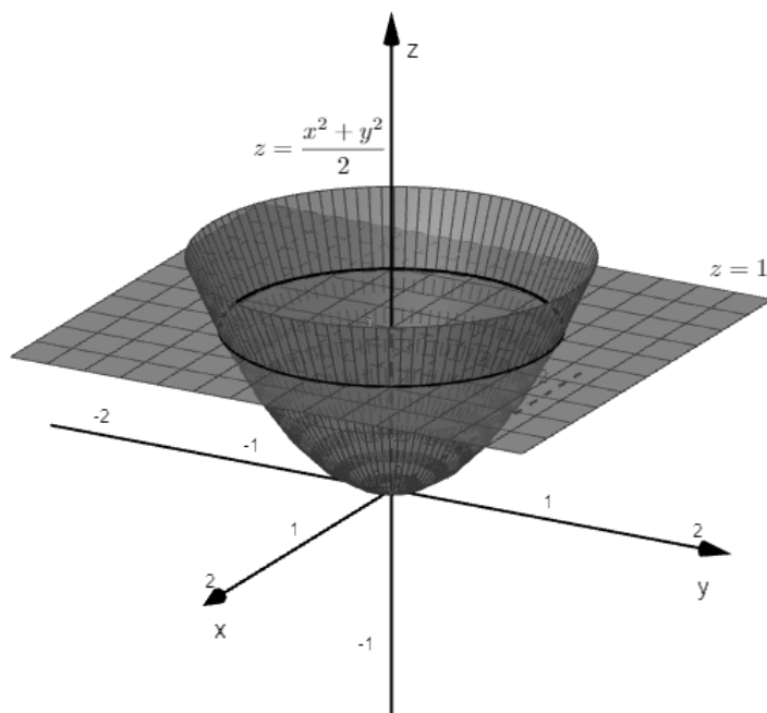
Slika 6.17: Ploha \Sigma
