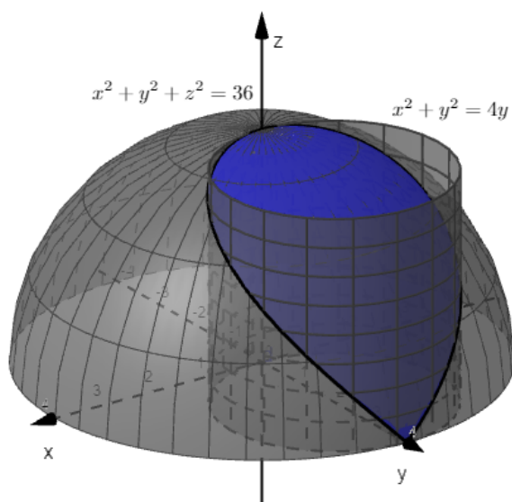
Slika 6.13: Ploha \Sigma
