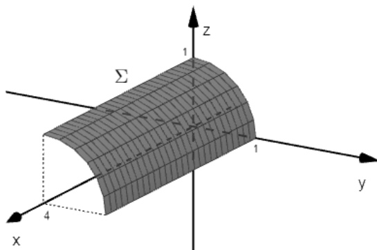
Slika 6.5: Ploha \Sigma
