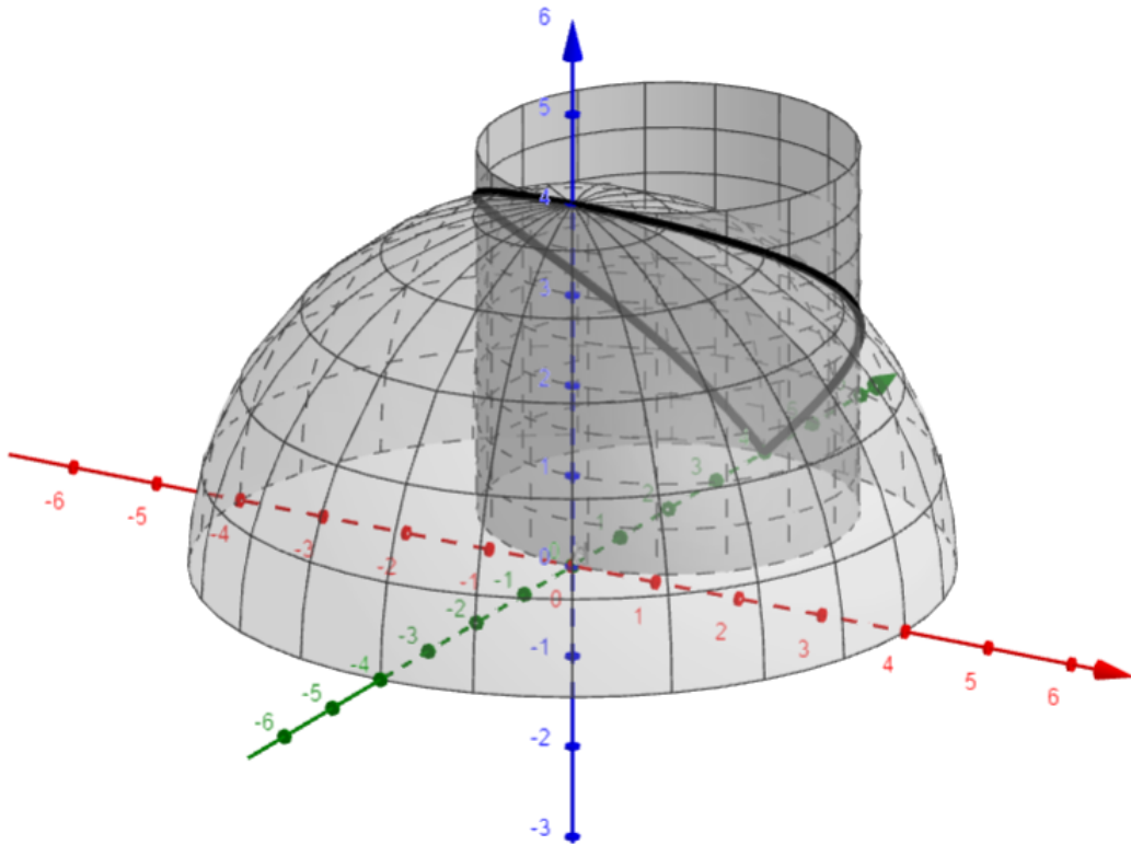
Slika 6.19: Ploha \Sigma
