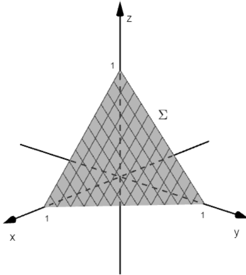
Slika 6.1: Ploha \Sigma
