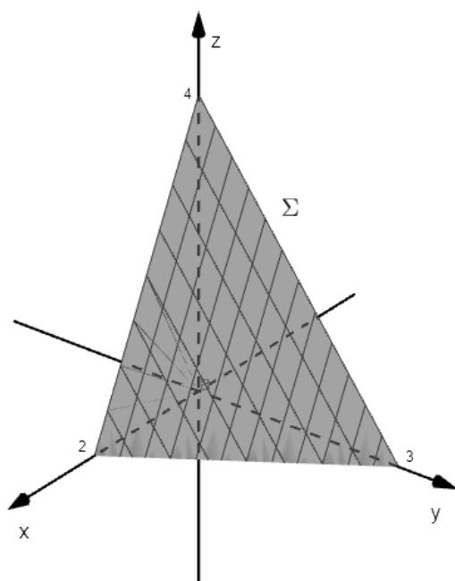
Slika 6.3: Ploha \Sigma
