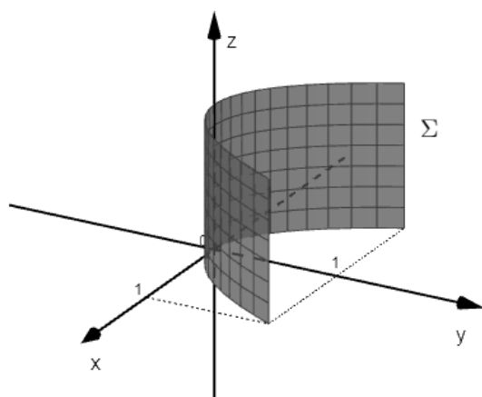
Slika 6.7: Ploha \Sigma
