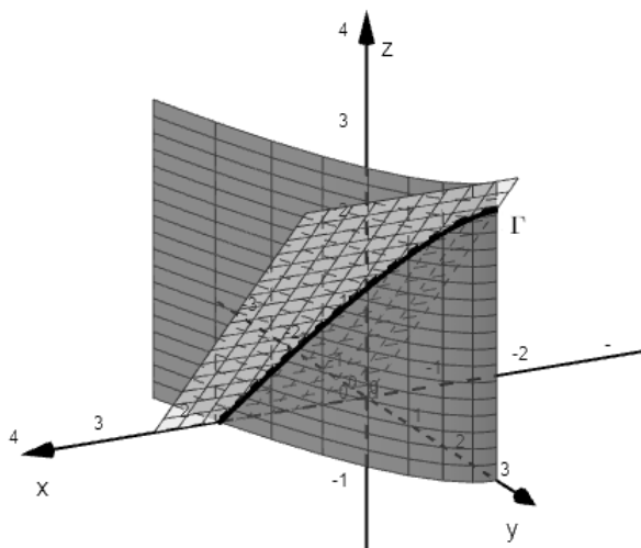
Slika 5.4: Krivulja \Gamma
