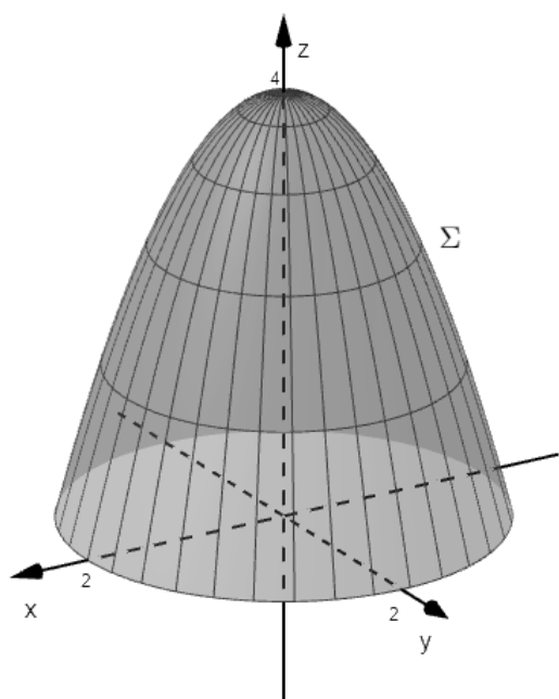
Slika 6.9: Ploha \Sigma
