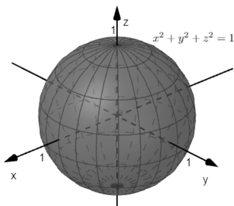
Slika 6.33: Ploha \vec{\Sigma}
