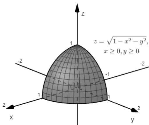
Slika 3.16: Tijelo \Omega
