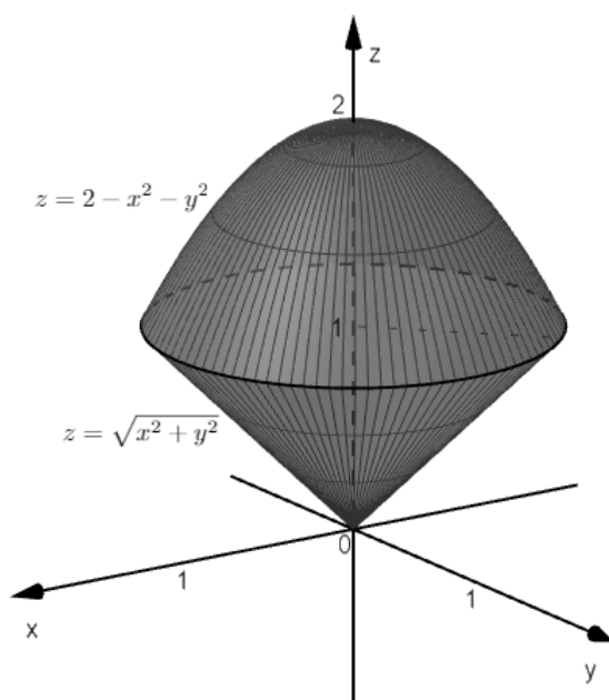
Slika 6.35: Ploha \vec{\Sigma}
