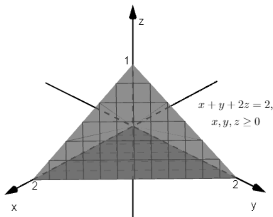
Slika 6.39: Ploha \vec{\Sigma}
