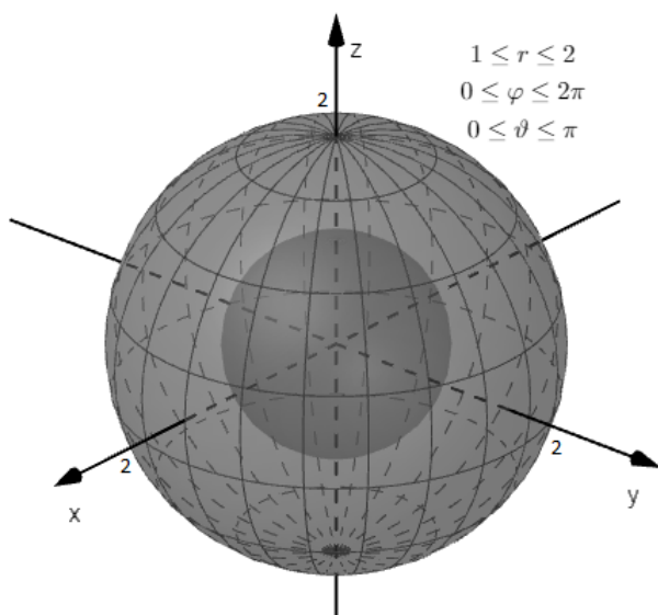
Slika 3.20: Područje integracije
