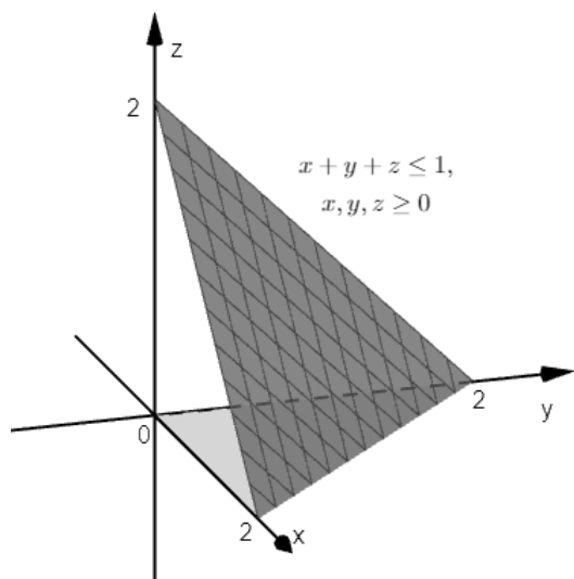
Slika 6.28: Ploha \vec{\Sigma}
