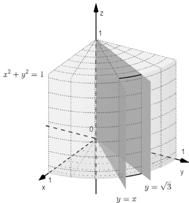
Slika 3.3: Tijelo \Omega
