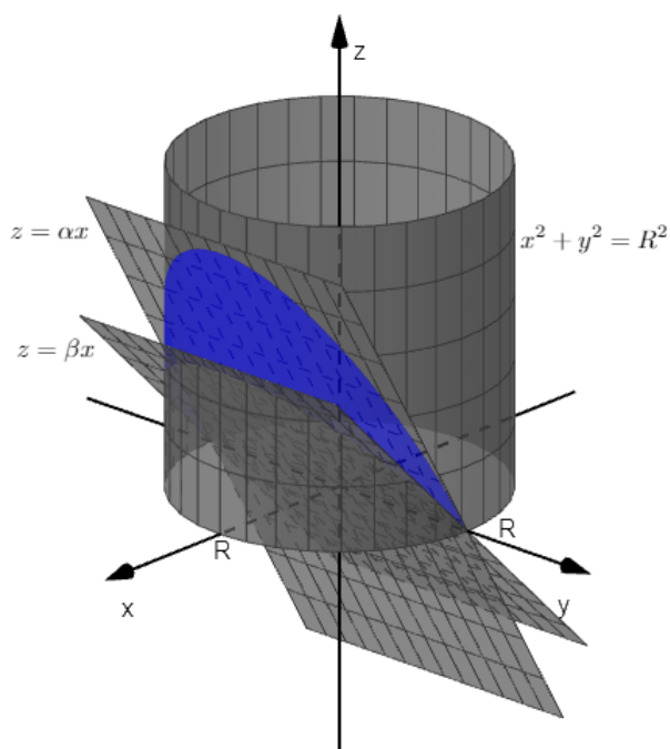
Slika 6.25: Ploha \Sigma
