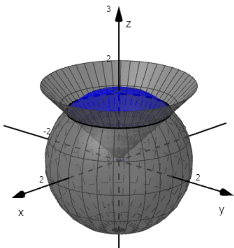
Slika 6.21: Ploha \Sigma
