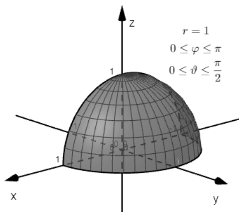
Slika 3.19: Područje integracije
