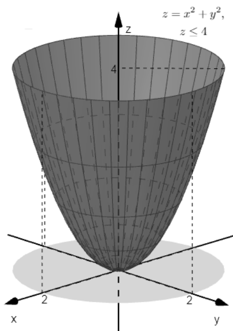
Slika 6.32: Ploha \vec{\Sigma}
