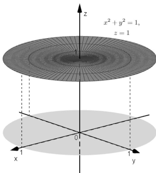
Slika 6.27: Ploha \vec{\Sigma}
