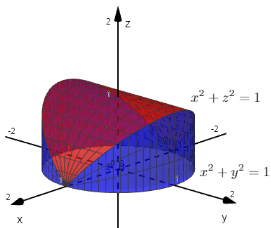
Slika 6.11: Ploha \Sigma
