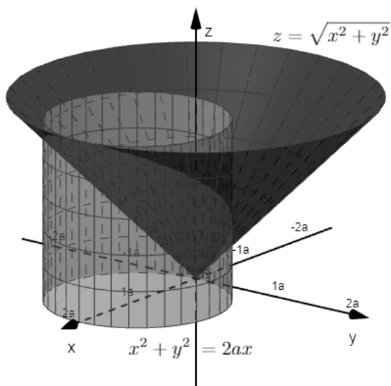
Slika 6.15: Ploha \Sigma
